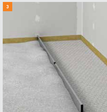
3 Srovnání voštinového zásypu fermacell
